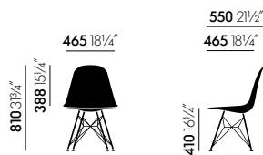
DSR, Drahtuntergestell mit Verstrebungen, nicht stapelbar, ohne Polster
